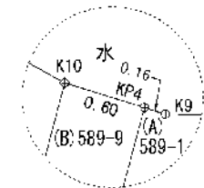
拡大図1 縮尺 1/50
